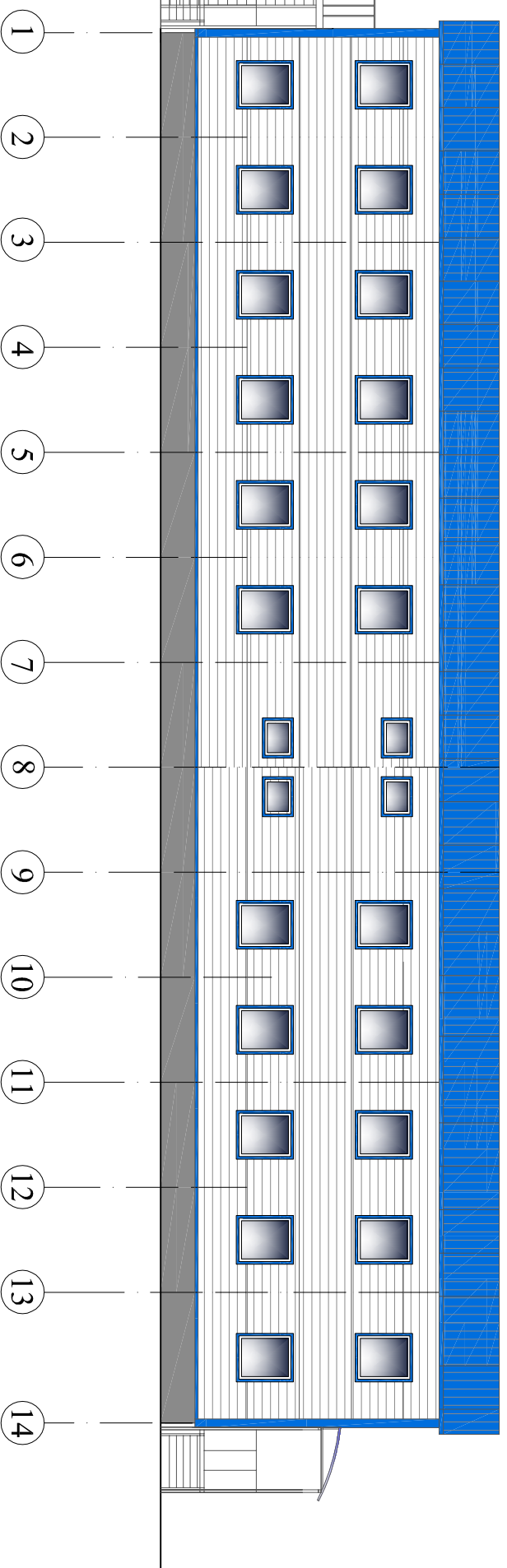
Фасад в осях 14 - 1
