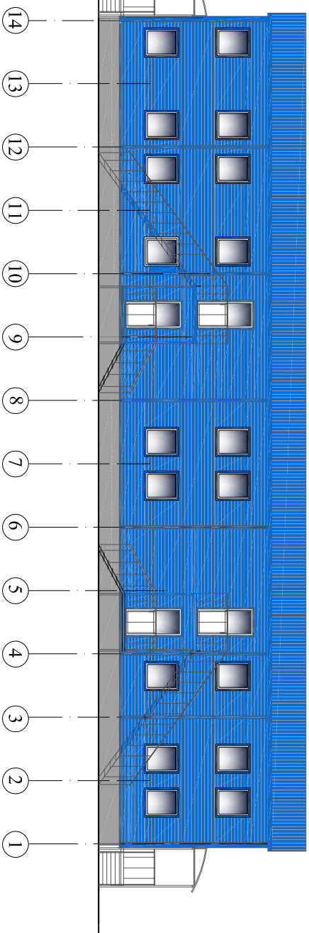
Фасад в осях 14 - 1
